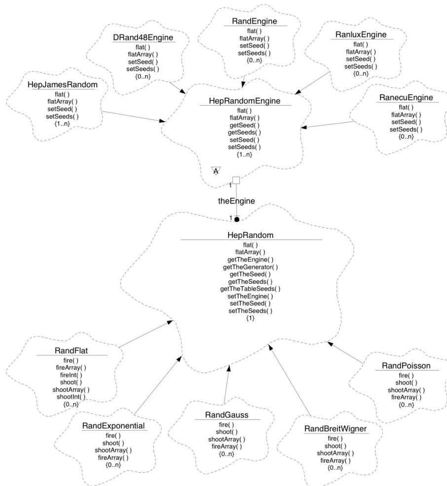
Fig. 2.24: HEPRandom module
