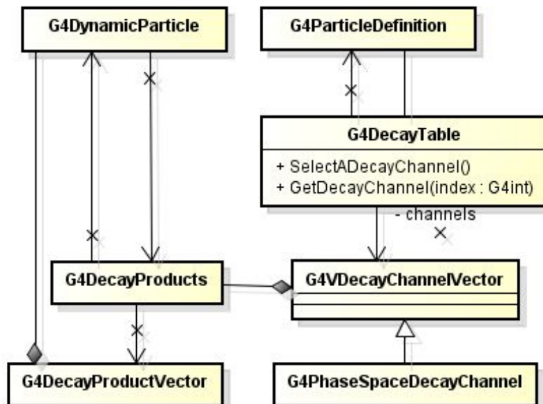
Fig. 2.20: Decay Table
